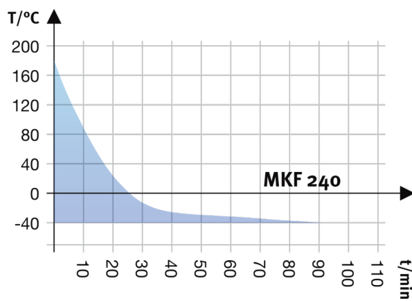
Abkühlkurve
