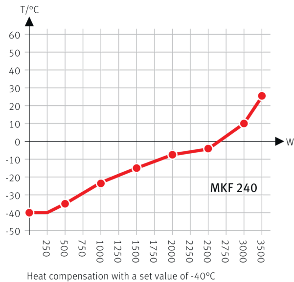
Wärmekompensationsdiagramm
